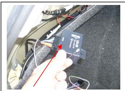
Anschluss 14-poliges Modul
