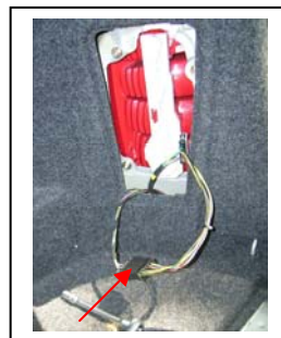
Anschluss Kabel Rückleuchte rechts
